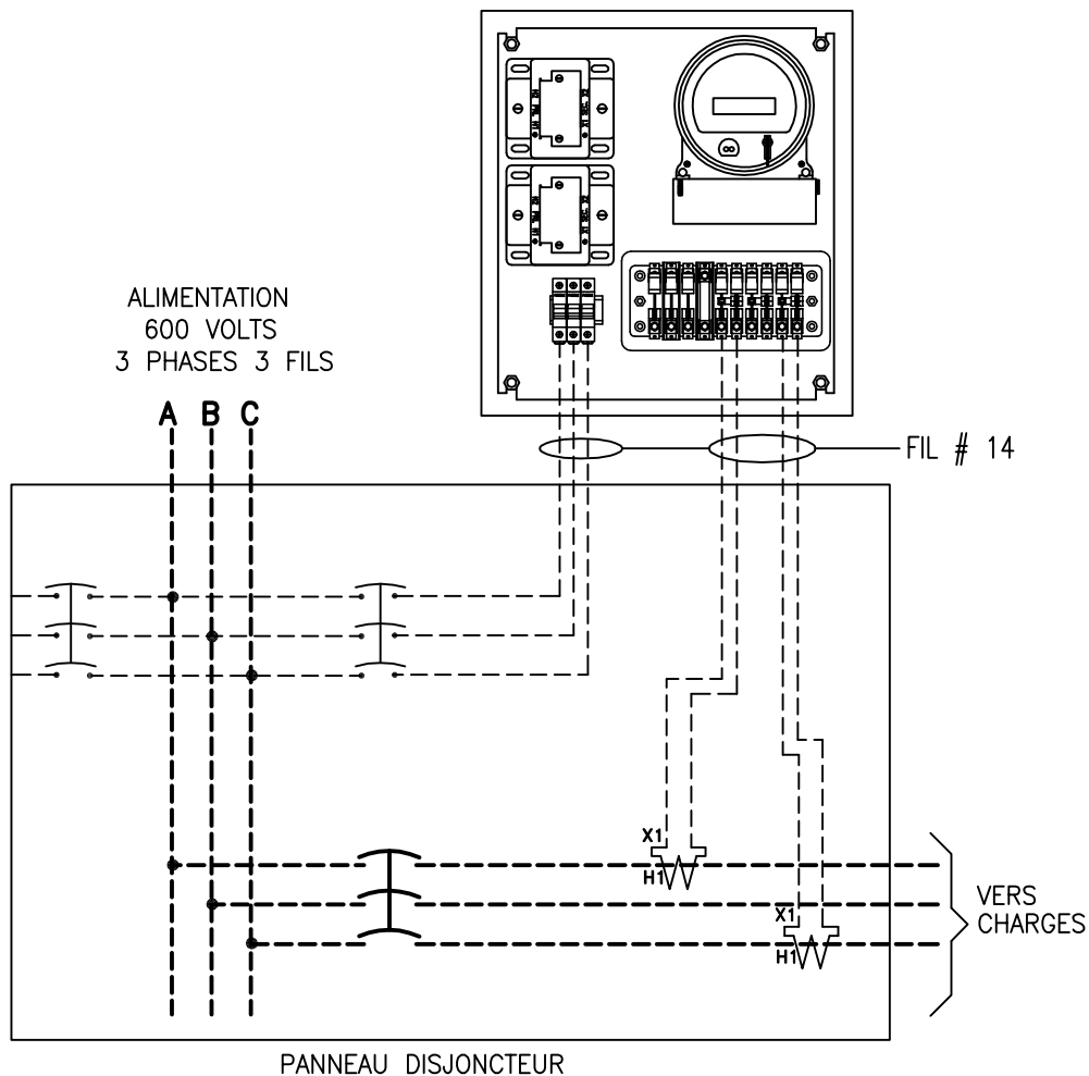
CABINET MESURAGE 20''x20''x8'' NEMA 1 VUE INTÉRIURE
